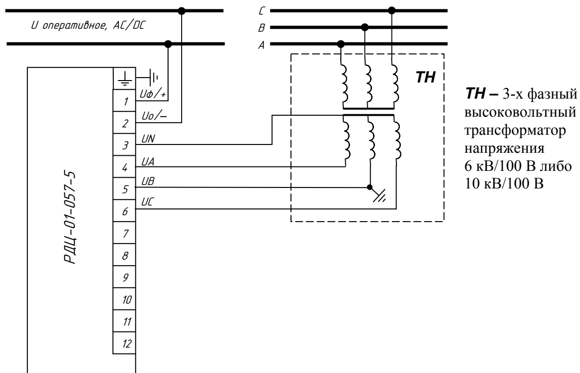
Рисунок 5 – Схема включения реле РДЦ-01-057-5 по напряжению
